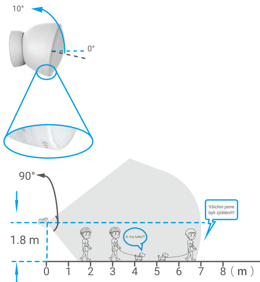
Obr. 1 Pohled z boku na rozsah detekce
