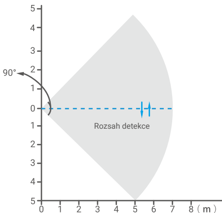
Obr. 2 Pohled shora na rozsah detekce
