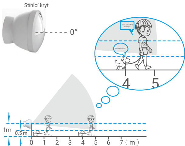
Obr. 1 Pohled z boku na rozsah detekce
