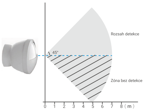
Obr. 2 Pohled shora na rozsah detekce
